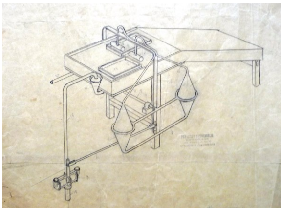
Macchina termo – solare
