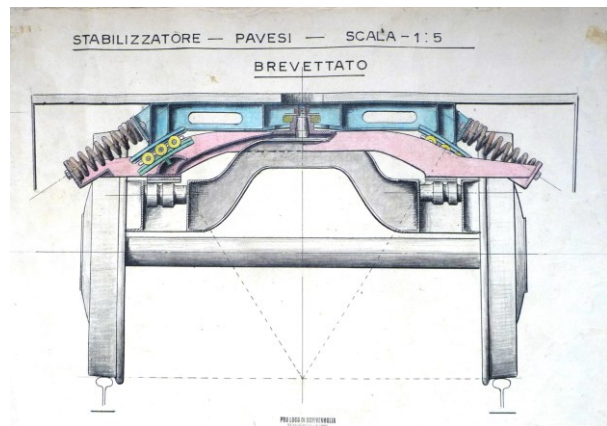
stabilizzatore ferroviario
